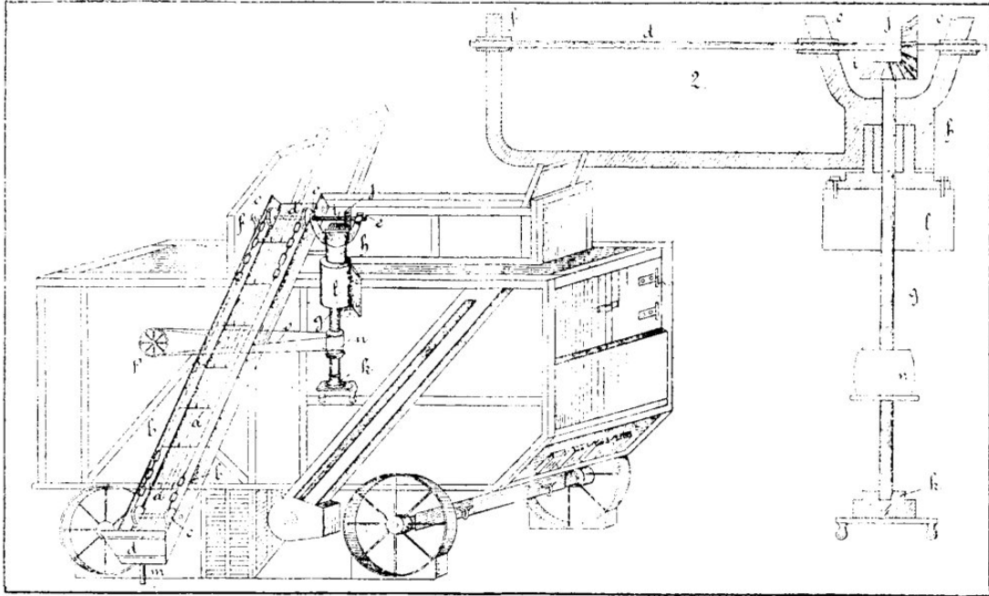
57. ábra. Kévehordó elevátor.
