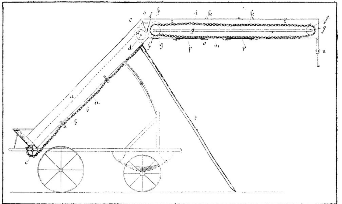
58. ábra. Kazalozó elevátor.
